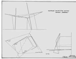
"vis à vis" [sic] Haltepunkte in der Landschaft, 1991 2-teilig Konstruktionszeichnung 1:20 Finleliner auf Papier Maße ?
